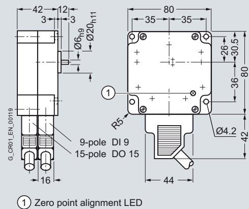
Opto-electronic encoder 6GA4 603-5AA00
